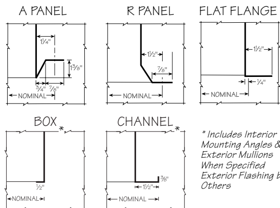
JAMB TYPES
