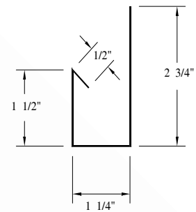
JAMB TRIM - JT17
